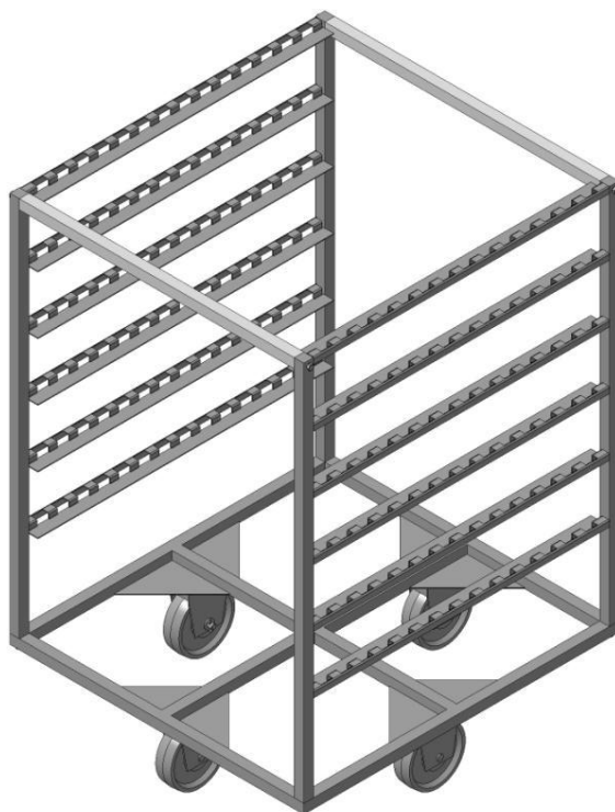
ТЕЛЕЖКА к КТД-100
